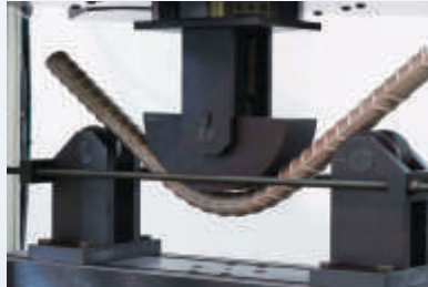
கம்பியை ISI முறையில் U வடிவில் வளைத்து அந்த வளைவில் வெடிப்பு, கிரிவு ஏதும் இல்லாமல் இருப்பதை வைத்து கம்பியின் தரத்தை கண்டறியலாம்.
